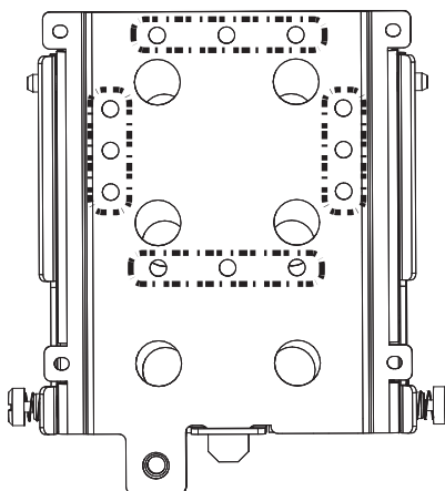
Fig. 3, Orificios de montaje para dispositivos Wi-Fi
