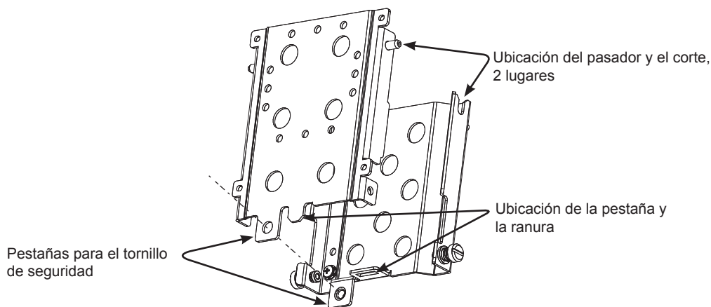
Fig. 4, Fijación de la placa superior a la placa inferior.
