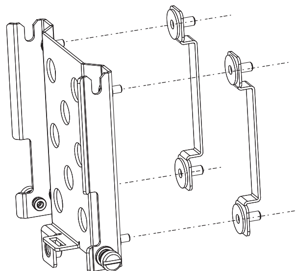
Fig. 2, Fijación de la base de la placa de montaje a las tiras interiores
