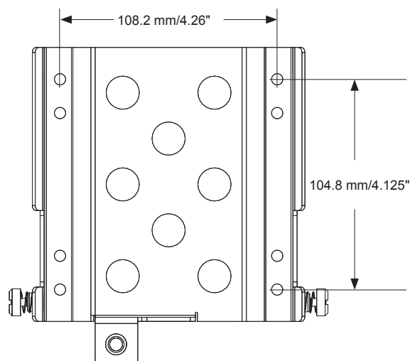
Fig. 1, Medidas de los orificios de montaje
